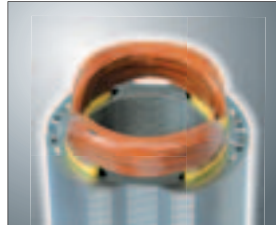
ラビリンス構造 粉じんが入りにくい。 モータ 防じんベアリング & 防じんワッシャ 粉じんの侵入をさらに防止。
