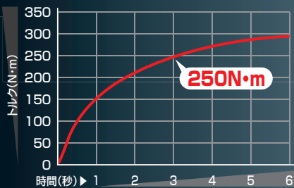
締付けトルクカーブ表 [高速時: M16高力ボルト、強度区分10.9]
